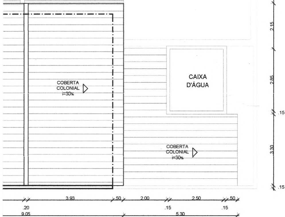
3 PLANTA DE COBERTURA ESCALA 1:100
