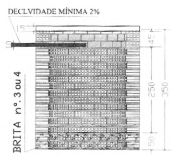
CORTE EE SUMIDOURO Esc.: 1:100
