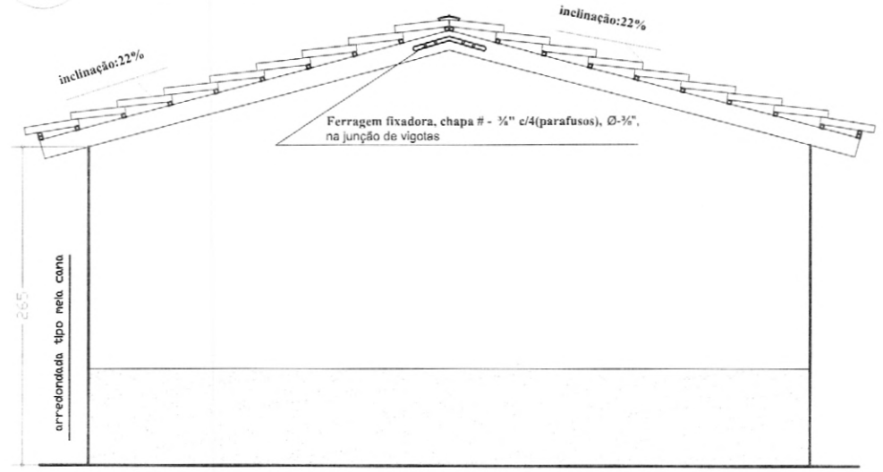
FACHADA LATERAL Esc. : 1 / 50
