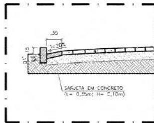
Detalhe - Sarjeta Sem Escala
