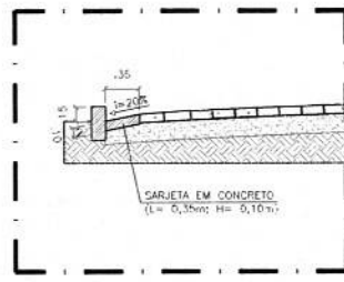
Detalhe - Sarjeta Sem Escala
