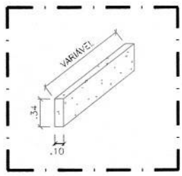
Detalhe - Banqueta Meio-Fio Sem Escala
