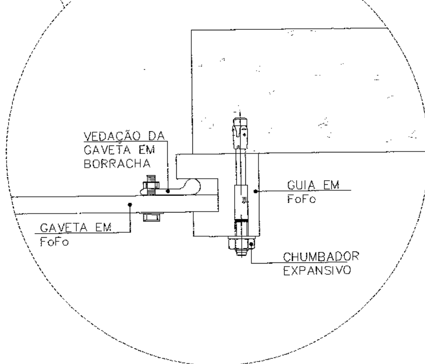
DETALHE DA COMPORTA SEM ESCALA
