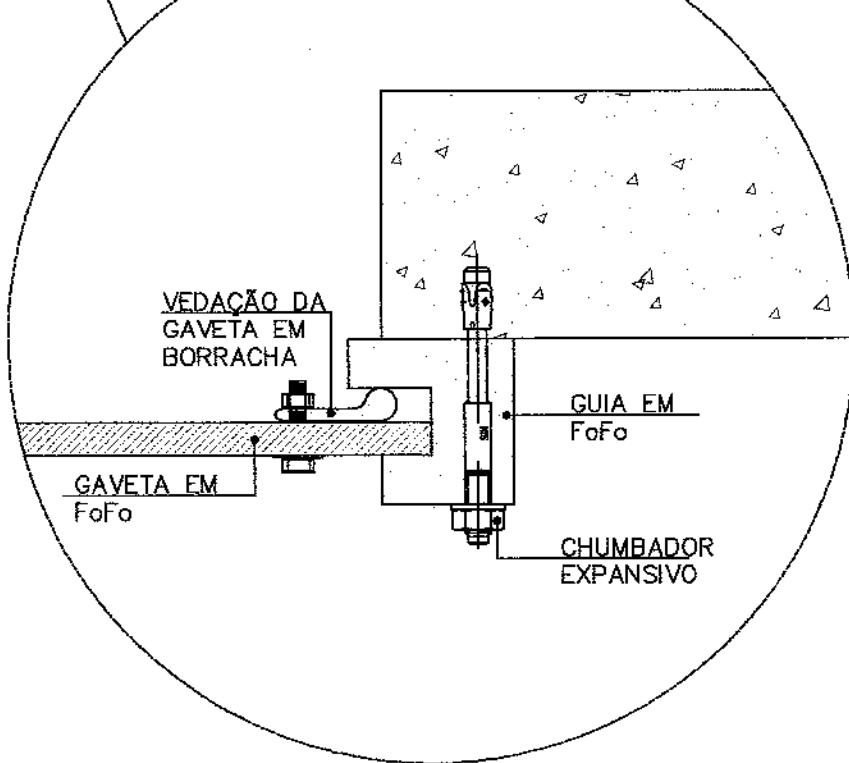
DETALHE DA COMPORTA SEM ESCALA
