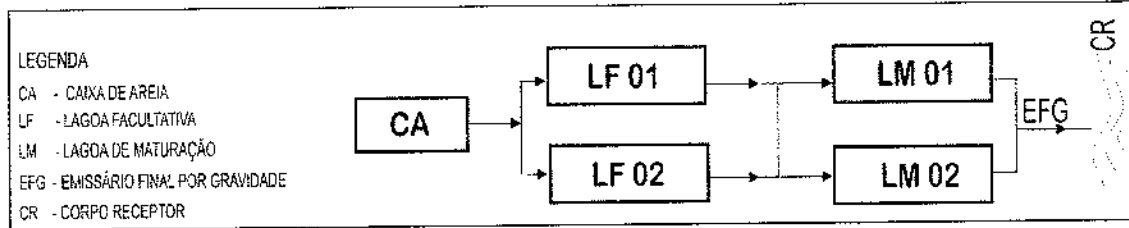
FIGURA 13 - CROQUI ESQUEMÁTICO DAS UNIDADES DA ETE
