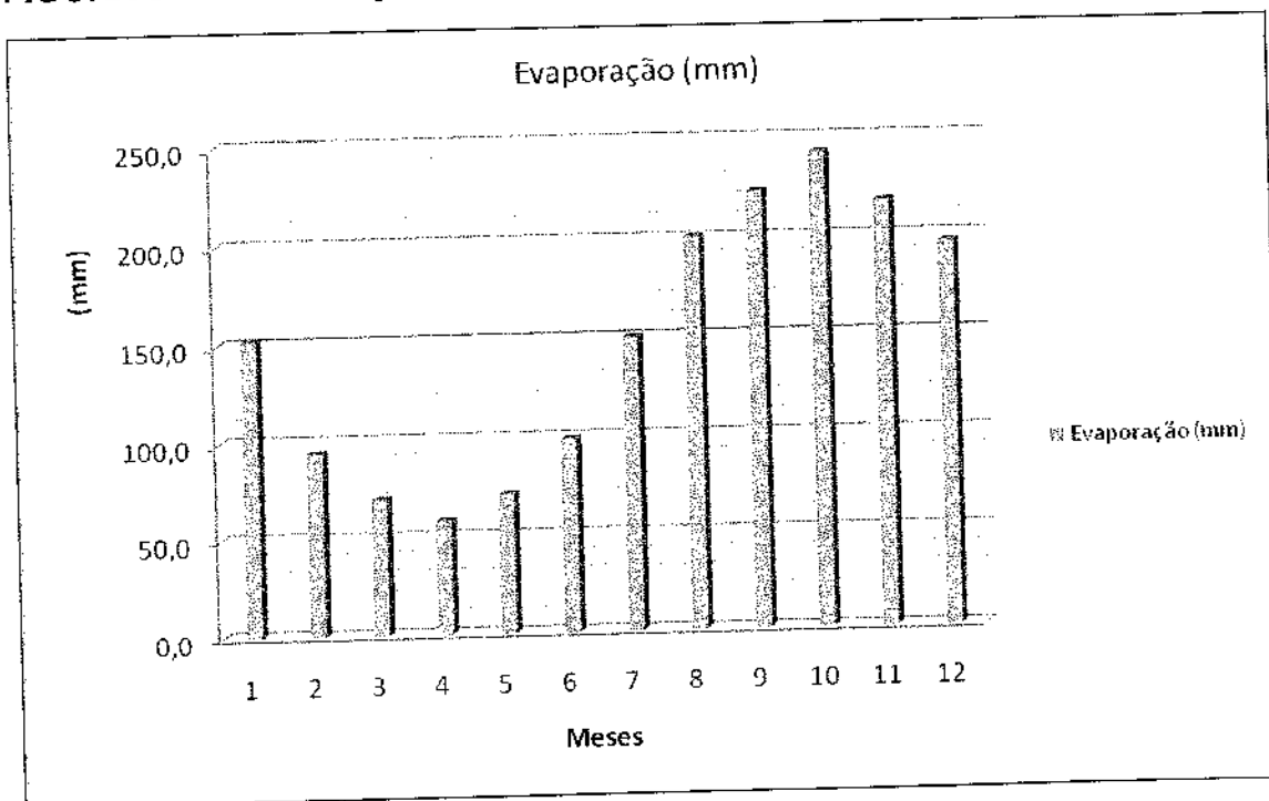
FIGURA 5 - EVAPORAÇÃO MÉDIA MENSAL (MM) EM SOBRAL - 1961 A 1990
