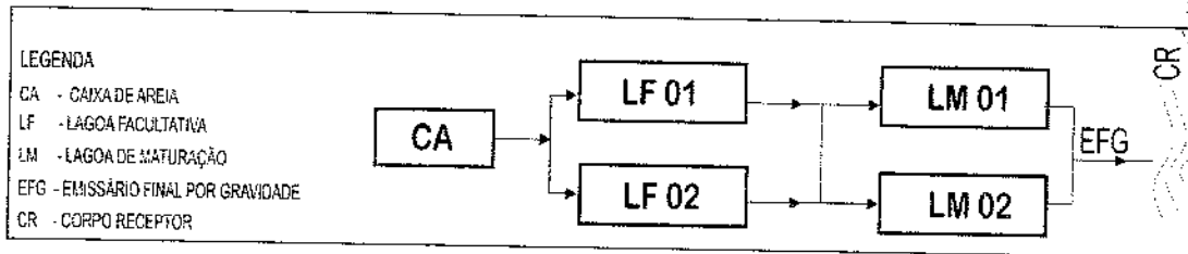
FIGURA 13 - CROQUI ESQUEMÁTICO DAS UNIDADES DA ETE – ETAPA FINAL
