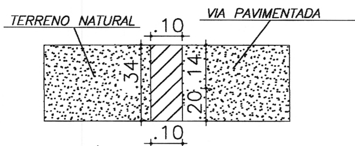
Detalhe do Meio-Fio Rebaixado Sem escala
