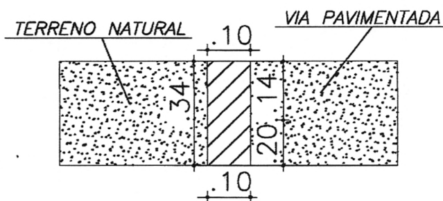
Detalhe do Meio-Fio Rebaixado Sem escala
