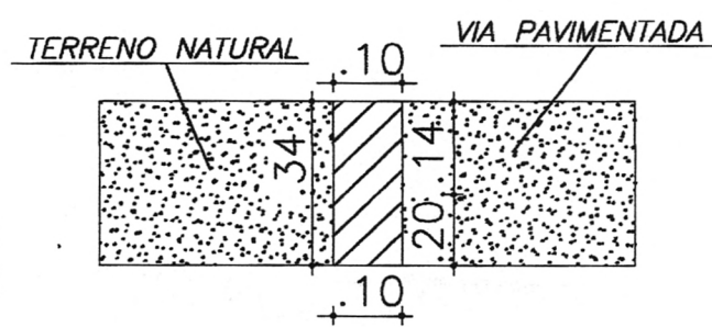
Detalhe do Meio-fio Rebaixado Sem escala
