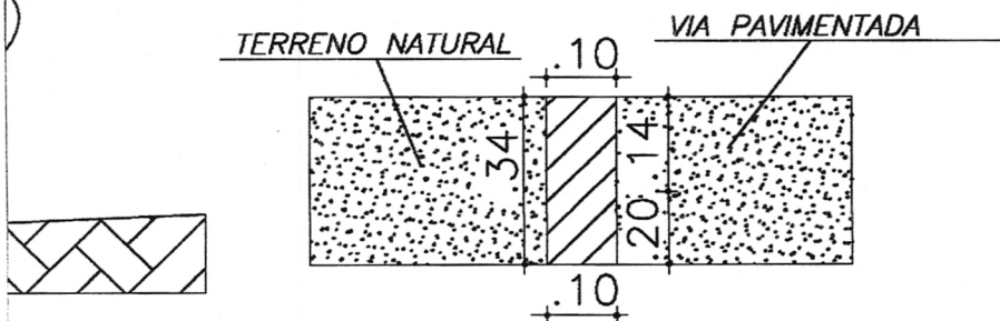
Detalhe do Meio-Fio Rebaixado Sem escala
