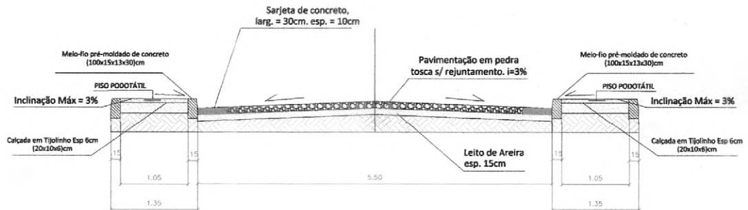
07 SEÇÃO TIPO DE PAVIMENTAÇÃO 5,50 m ESCALA: SEM ESCALA
