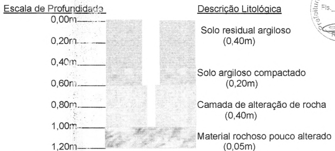
Fig. 09: Perfil Geológico esquemático em ST 04, Profundidade alcançada de 1,00m.
