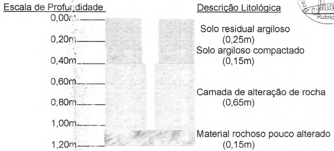
Fig. 06: Perfil Geológico esquemático em ST 07, Profundidade alcançada de 1,05m.
