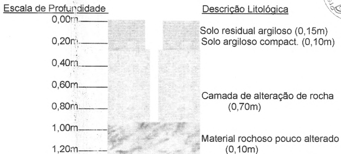
Fig. 10. Perfil Geológico esquemático ST 02 com Profundidade alcançada de 0,95m.
