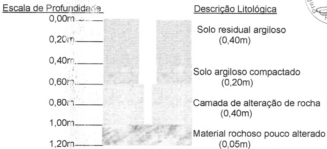
Fig. 13: Perfil Geológico esquemático, ST 16 com Profundidade alcançada 1,00m.
