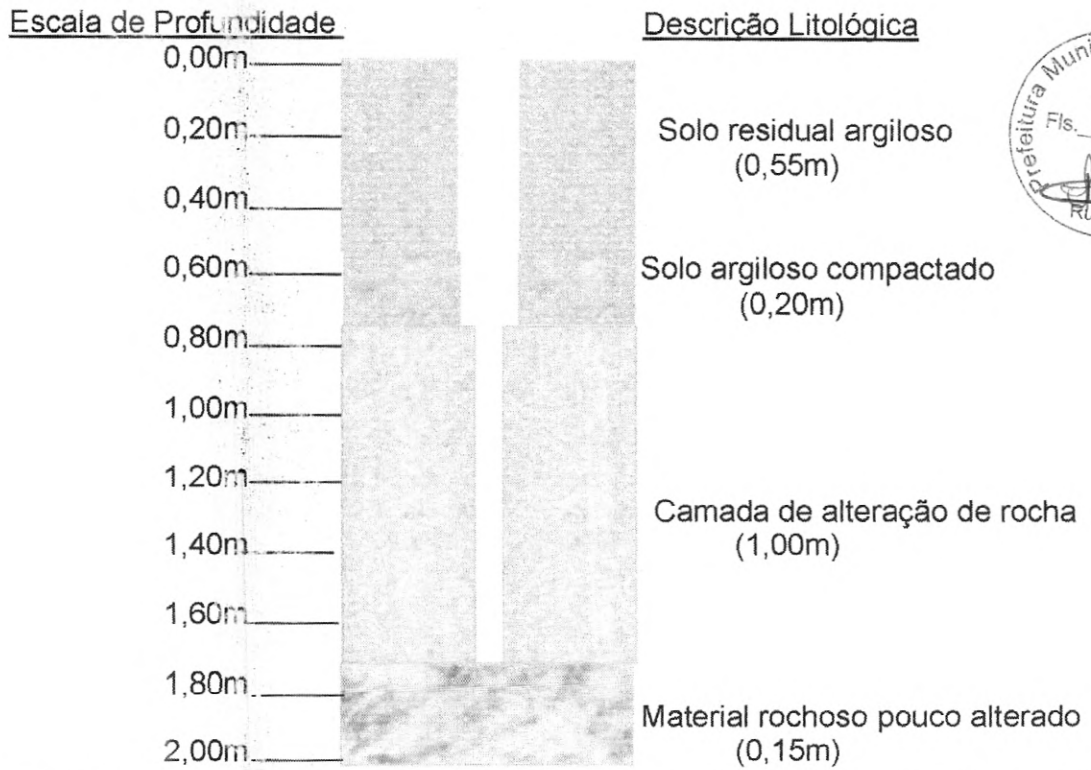
Fig. 03. Perfil Geológico esquemático em ST 05, Profundidade alcançada de 1,75m.
